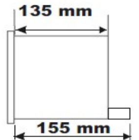
YANDAN GÖRÜNÜM
